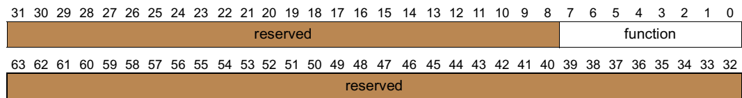
Figure 11-16. SALE_ENTRY State Parameter
