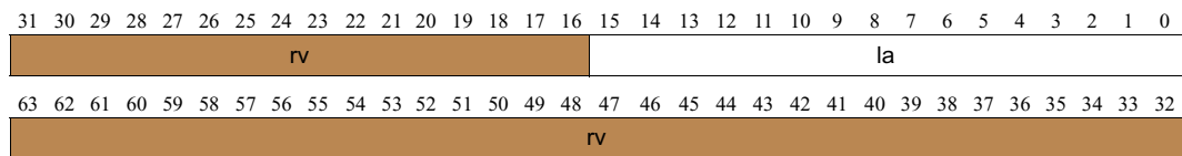
Figure 11-27. Layout of proc_n_log_info2 Return Value
