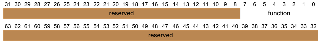
Figure 11-14. SALE_ENTRY State Parameter
