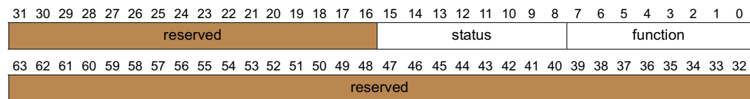
Figure 11-8. SALE_ENTRY State Parameter
